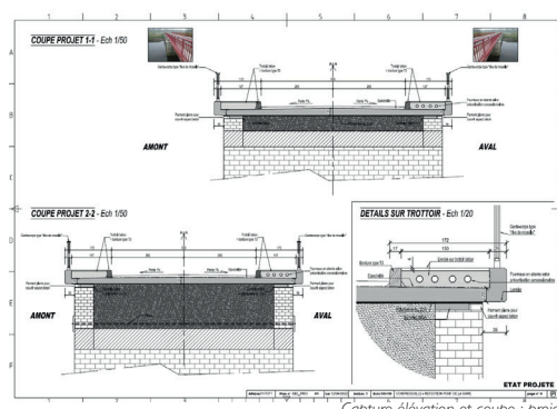
Capture élévation et coupe : projet
